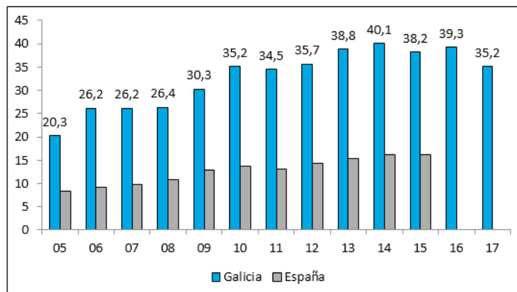
Gráfico 51. Evolución do consumo final bruto de enerxía procedente de FER (%)
