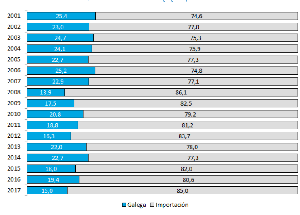
Gráfico 50. Evolución da Enerxía primaria galega e importada 2001-2017
