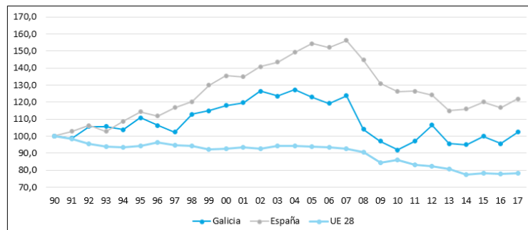
Gráfico 53. Evolución índice emisión GEI Galicia-España-Europa 1990-2017. (1990=100)
